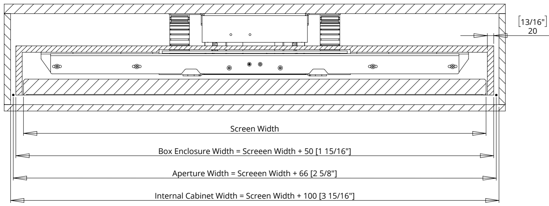
SECTION B-B SCALE 1 : 7
